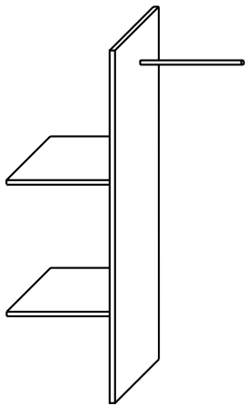
Mittelwandensatz, steingrau , inklusive 2 Einlegeböden und einer Kleiderstange, Maße: B/H/T 88/147/45 cm Art.-Nr. 499789
