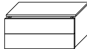
Schubkasteneinsatz, steingrau , 2 Schübe, Maße: B/H/T 88/39/45 cm Art.-Nr. 499803
